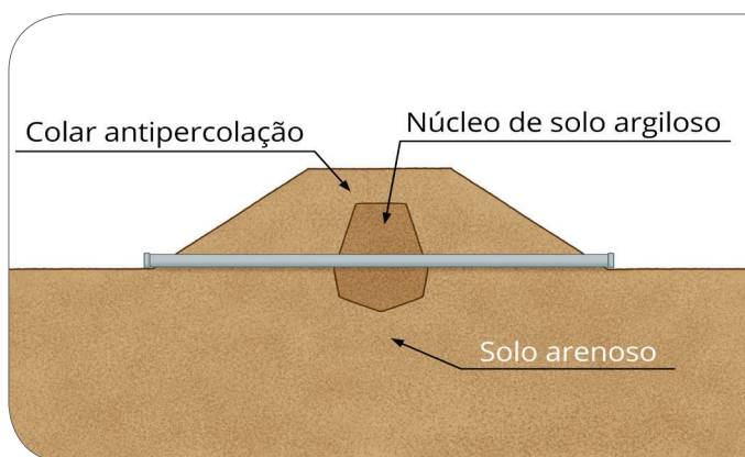
Corte de um talude com núcleo argiloso
