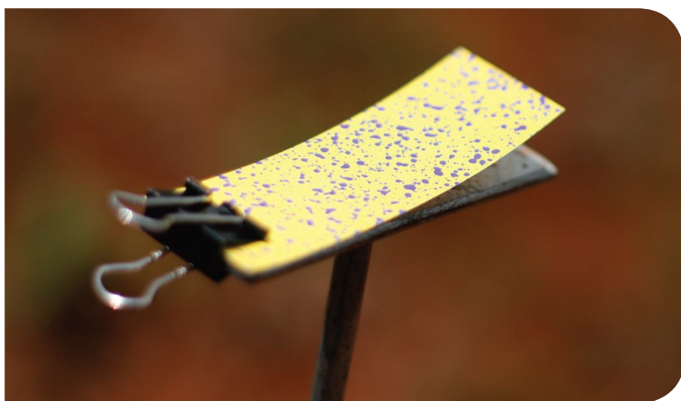
Papel hidrossensível mostrando gotas de tamanho uniforme
