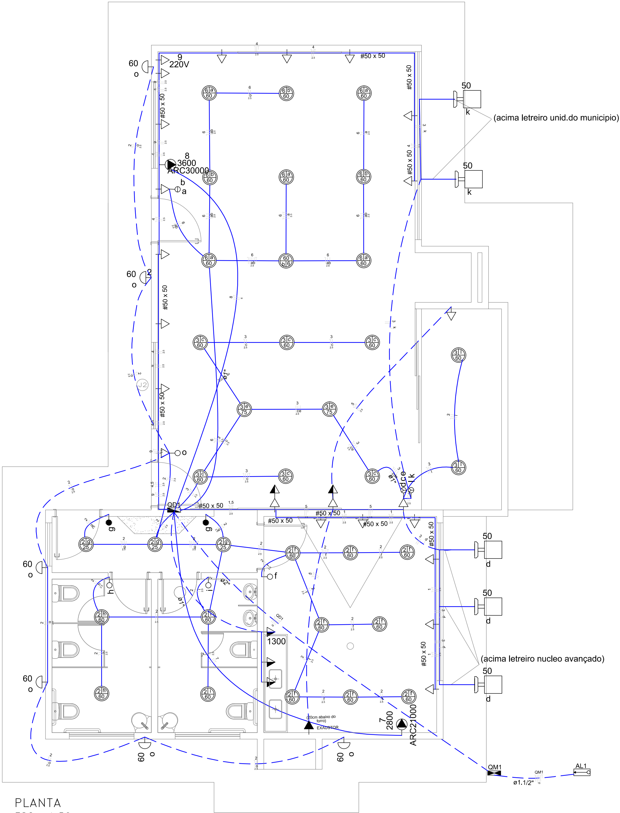
PLANTA ESC.: 1:50
