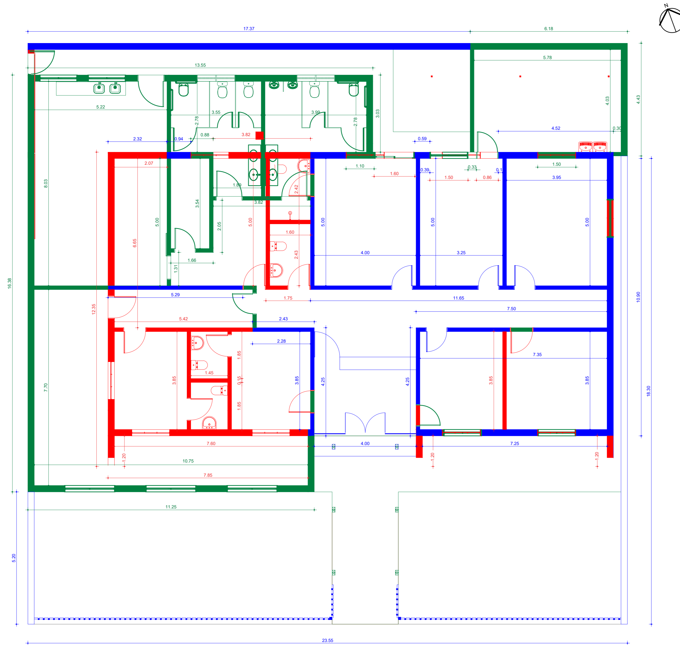
1 PLANTA BAIXA - CONSTRUIR / DEMOLIR 1:75
