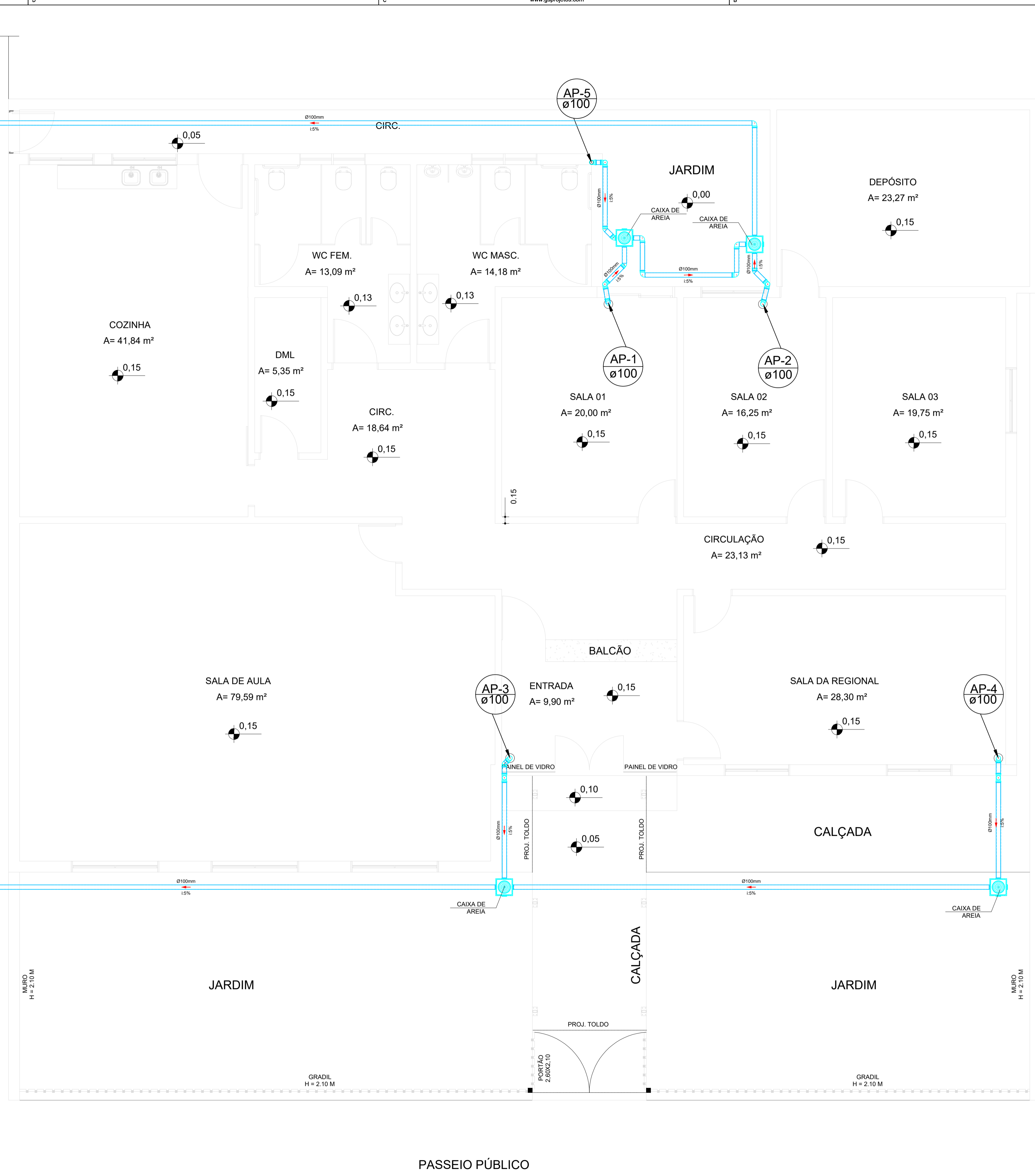
1 PLANTA BAIXA 1:50
