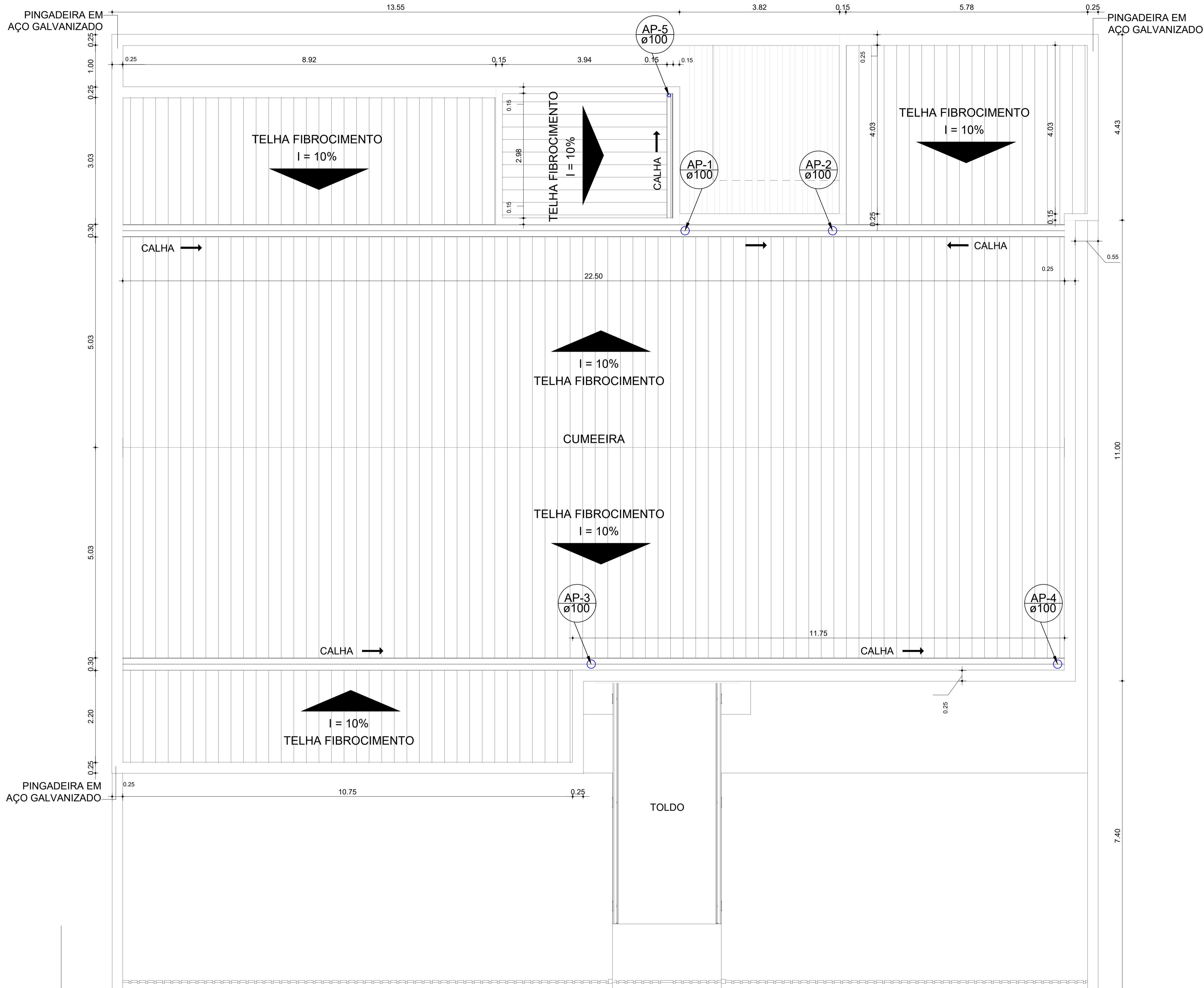
1 PLANTA DE COBERTURA 1:50
