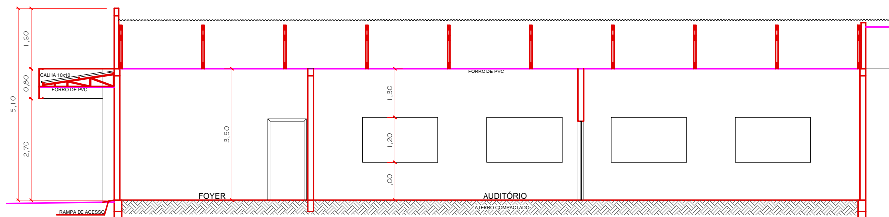
01 CORTE BB ESC. 1/100
